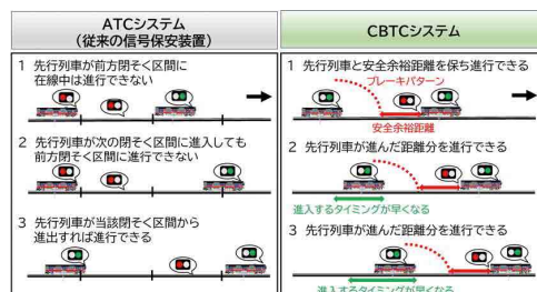
丸ノ内線CBTCシステム
