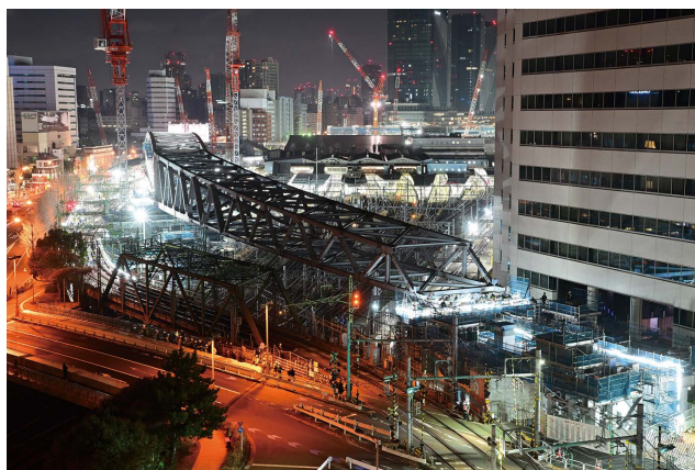
連続立体交差化工事(京急本線)
